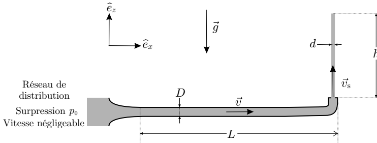
FIGURE 5 – Jet d'eau vertical
