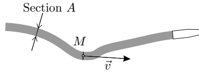
FIGURE 2 – Lance à incendie
