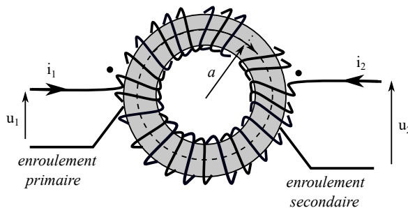
FIGURE 7 – Transformateur
