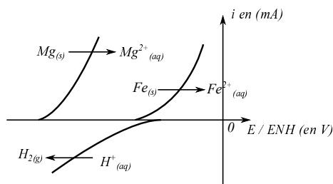
FIGURE 11 – Courbes intensité - potentiel
