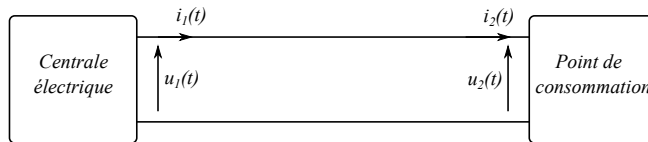
FIGURE 9 – Distribution de l'énergie électrique
