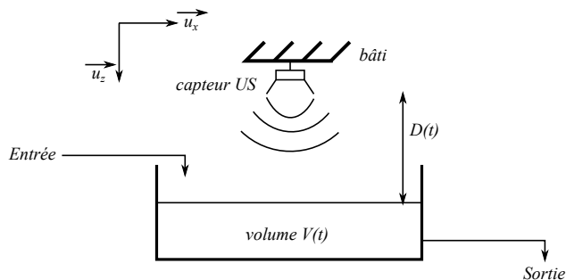
FIGURE 2 – Bassin et capteur à ultrasons
