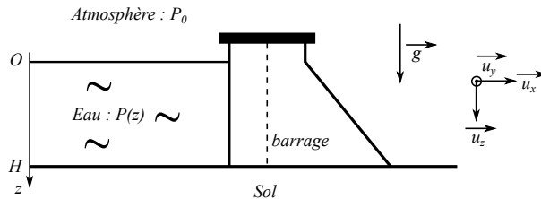
FIGURE 1 – Un barrage poids de forme trapézoïdale
