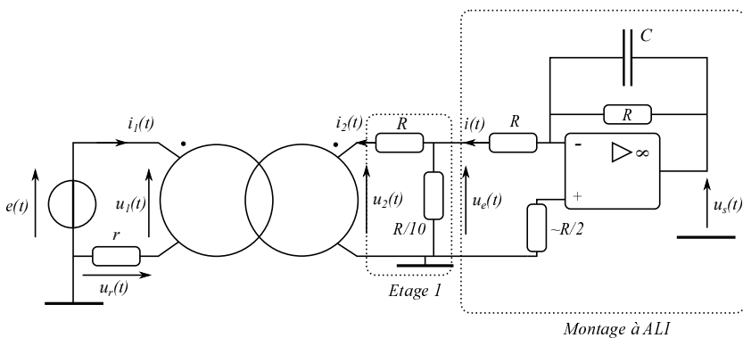
FIGURE 8 – Schéma du montage réalisé
