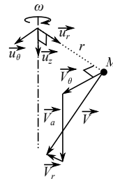
Décomposition cylindrique
