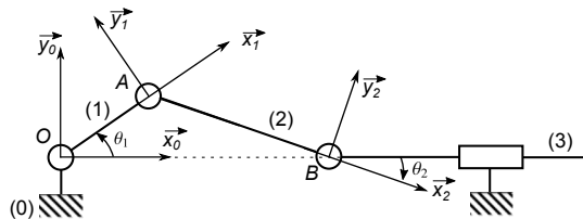
Figure 2 - Schéma cinématique d'une partie de la pompe
