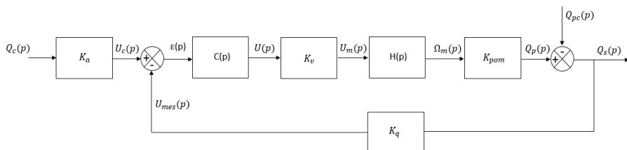
Figure 4 - Schéma-bloc de l'asservissement du débit
