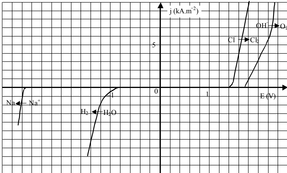
Figure 13 - Courbes intensité-potentiel sur une électrode de tungstène
