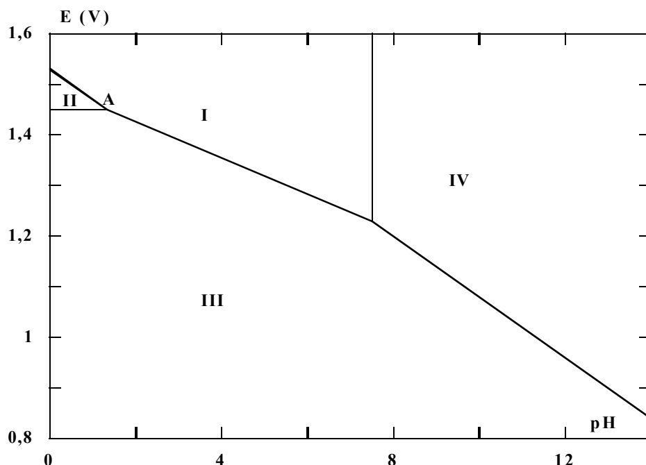
Figure 5 - Diagramme de Pourbaix du chlore
