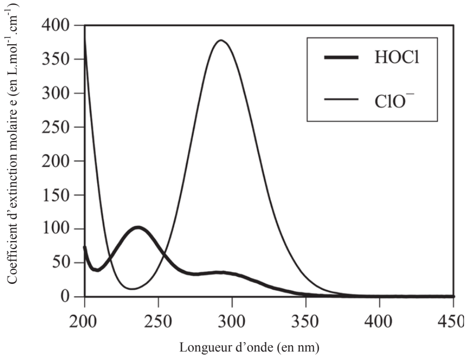
Figure 7 - Courbe d'extinction molaire des espèces chlorées considérées
