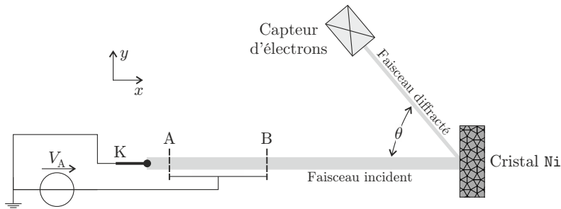
FIGURE 5 – Schéma de l'expérience de DAVISSON et GERMER, 1927
