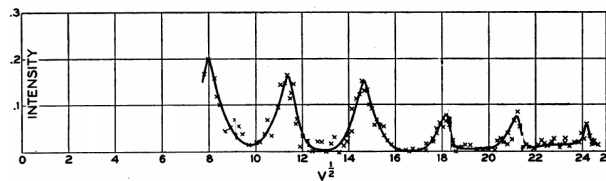
FIGURE 7 – D'après Davison et Germer, Proc. Nat. Acad. Sci. USA , 1928
