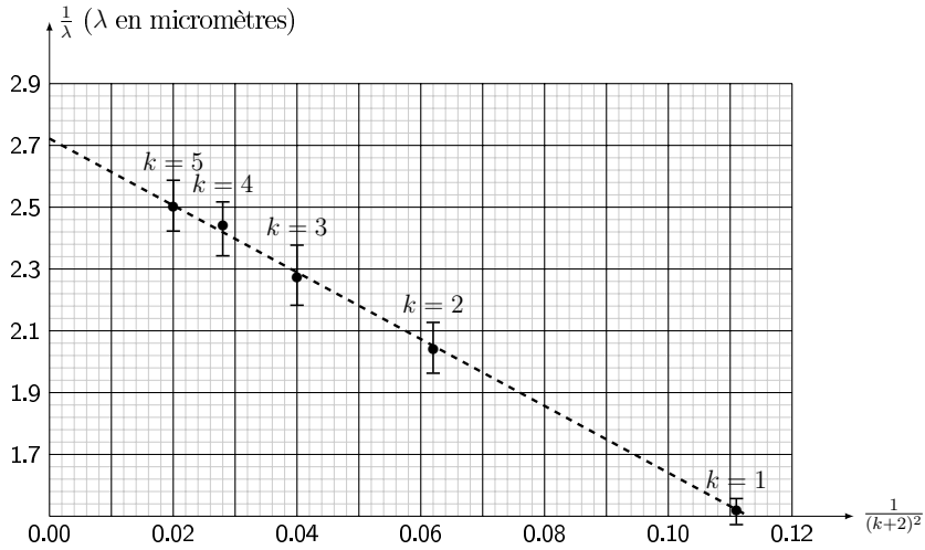
FIGURE 1 – Tracé de 1/\lambda_0 en fonction de 1/(k+2)^2
