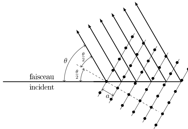
FIGURE 6 – Réseau de plans réfléchissant le faisceau d'électrons
