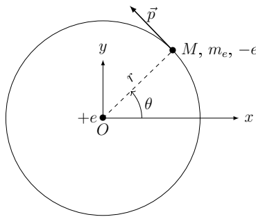
FIGURE 2 – Modèle de BOHR pour l'atome d'hydrogène
