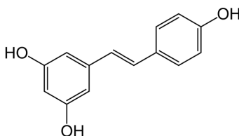
FIGURE 1 – Structure du resvératrol
