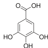
FIGURE 2 – Structure de l'acide gallique
