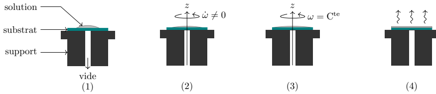
Figure 4 – Étapes de la procédure d'enduction centrifuge.
