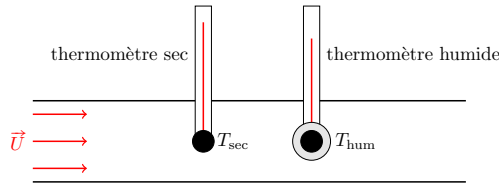
Figure 3 – Psychromètre.
