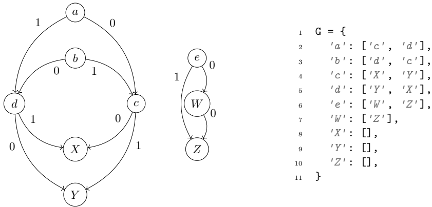
FIGURE 1 – Exemple de graphe avec sa représentation Python.
