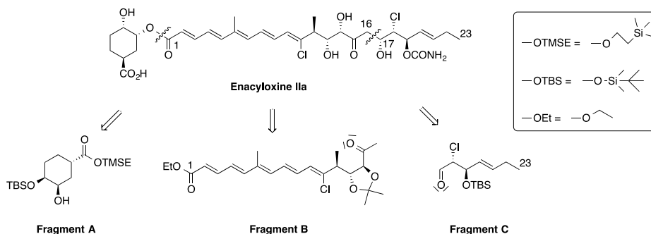
Figure 7 : Analyse rétrosynthétique de l'énacyloxine IIa
