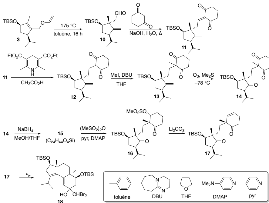
Schéma 3. Obtention du composé 18 .
