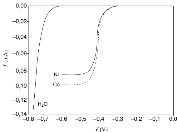
Figure 6. Courbes courant-potentiel.
