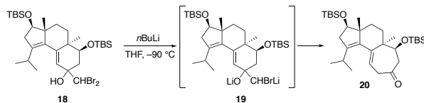
Schéma 4. Formation du cycle à sept chaînons de la cynréine A par expansion de cycle.
