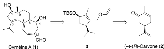
Schéma 1. Synthèse de la cynréine A à partir de la (–)-(R)-carvone.
