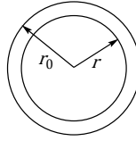
Figure 1. Modèle de particule sphérique solide.
