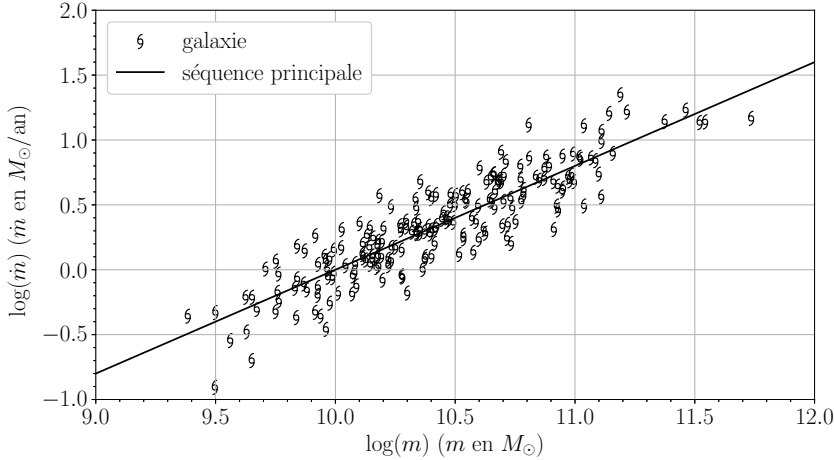
FIGURE 6 – Séquence principale des galaxies
