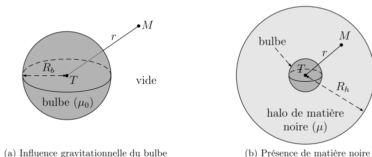
FIGURE 5 – Modèles galactiques
