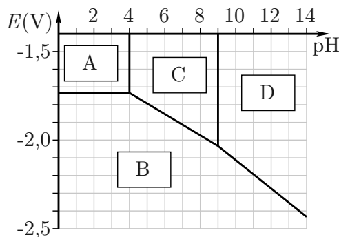
Figure 7 – Diagramme potentiel-pH de l'aluminium
