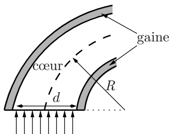
Figure 6 – Fibre optique courbée
