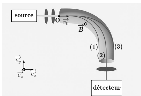
Figure 2 – Schéma de principe du spectromètre de masse
