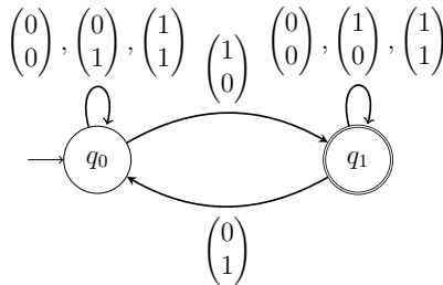
FIGURE 2 – Représentation de l'automate \mathcal{A}_2
