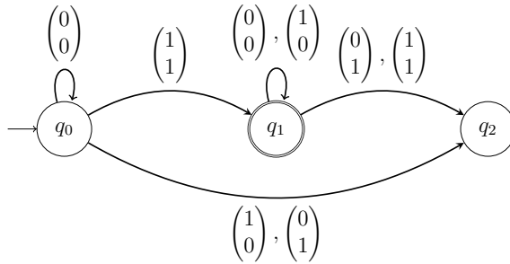
FIGURE 1 – Représentation de l'automate \mathcal{A}_1
