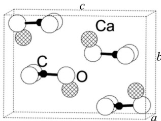
Figure 8 – Représentation de la maille de l'aragonite.
