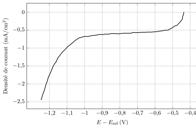
Figure 7 – Courbe courant/potentiel cathodique pour une électrode d'acier.
