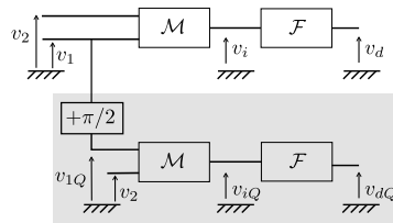
Figure 5 – Principe d'un montage de détection synchrone.
