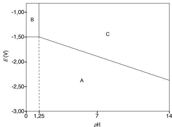
Figure 1. Diagramme E-pH du zirconium.
