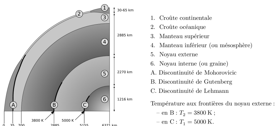
Figure 1 Structure de la Terre. D'après Wikipédia.
