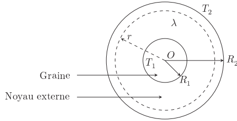
Figure 7 Schématisation du noyau terrestre.
