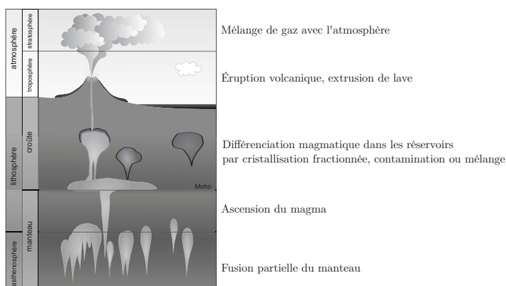
Figure 8 Magnétisme et volcanisme. D'après Wikipédia.
