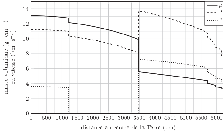
Figure 3 Profils de la masse volumique et des vitesses des ondes P et S dans le modèle PREM. D'après Dziewonski A. M., Anderson D. L., 1981. Preliminary reference Earth model . Physics of the Earth and Planetary Interiors. Vol. 25, n° 4, p. 297-356.
