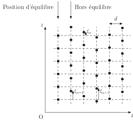
Figure 2 Représentation schématique des déplacements atomiques.
