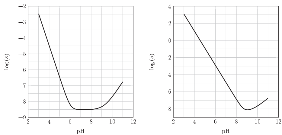
Figure 11 Diagramme de solubilité de l'espèce \text{NiO(s)} en fonction du pH pour deux températures : 300 °C et 90 °C.
