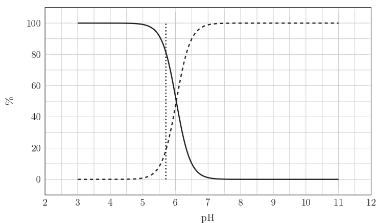
Figure 10 Diagramme de distribution à 300 °C.
