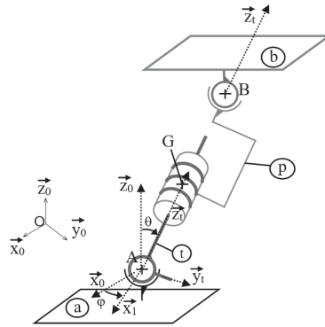
FIGURE 4 – Modèle cinématique du robot Delthaptic.
