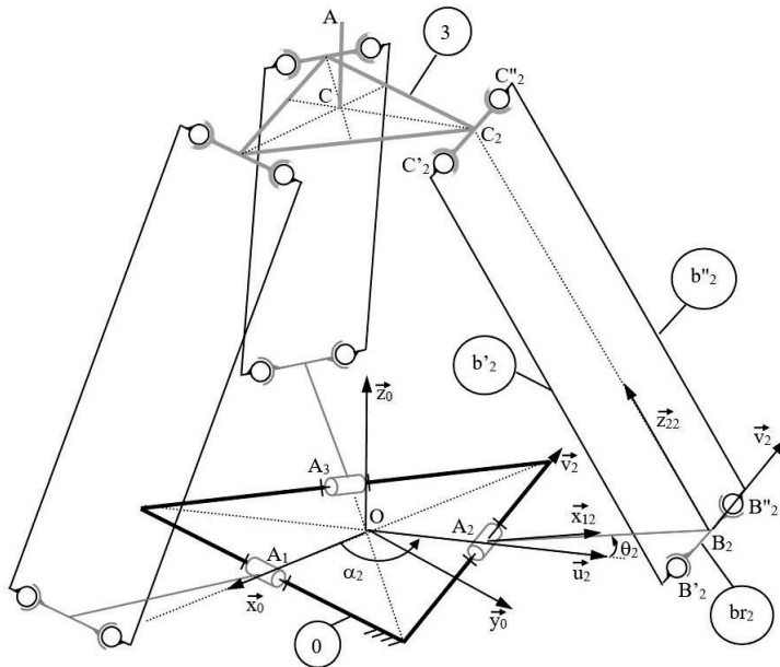
FIGURE 2 – Modèle cinématique d'un robot Delta.
