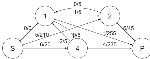
Figure 11 - Exemple d'extrait de graphe avec flot
