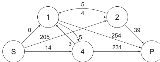
Figure 12 - Exemple de graphe résiduel
