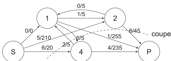
Figure 13 - Coupe dans un graphe
