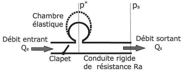
FIGURE 16 – Schéma du modèle de Windkessel
