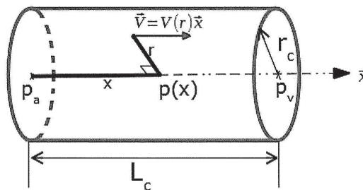
FIGURE 14 – Écoulement de Poiseuille dans un tube cylindrique
