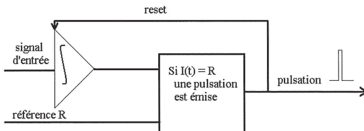
FIGURE 25 – Schéma de principe du générateur d'impulsions.
