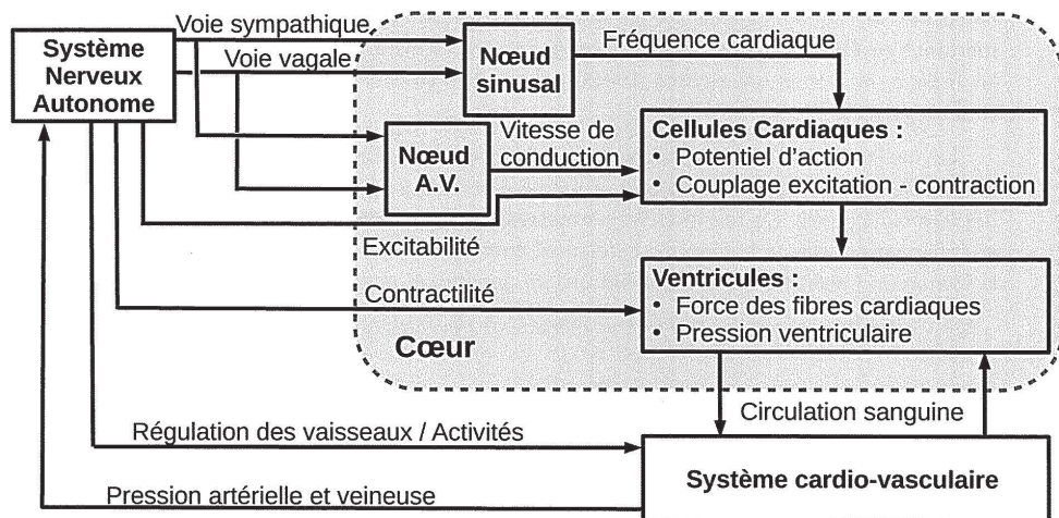
FIGURE 3 – schéma de principe de la régulation sanguine
