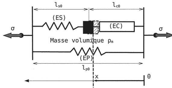
FIGURE 9 – Modèle massique de Maxwell Hill
