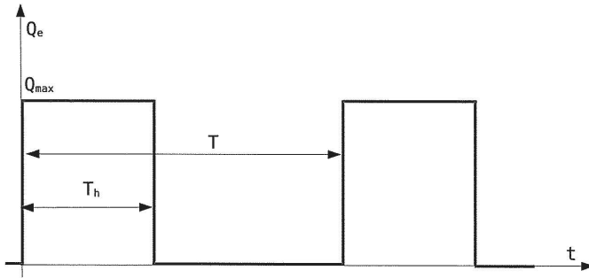
FIGURE 17 – Approximation en signal crêteau du débit sortant du cœur
