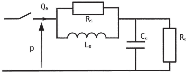
FIGURE 18 – Modèle de Windkessel à 4 éléments
