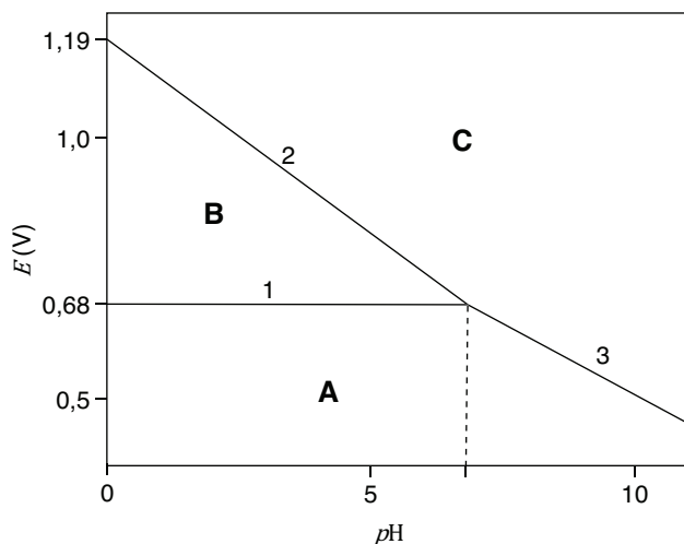
Figure 2. Diagramme potentiel- p\text{H} de quelques espèces de l'iode.
