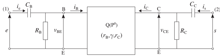
FIGURE 13 – Modèle “petit signal” de la structure amplificatrice complète constituée du transistor et de son environnement électrique.
