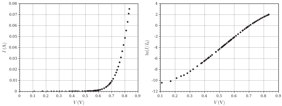
FIGURE 8 – Caractéristique expérimentale I = I(V) d'une diode 1N4148 (pour T = T_a et V \geq 0 (V)). L'axe des ordonnées du tracé de droite porte le logarithme népérien du rapport I/I_0 où I_0 est un courant de référence.
