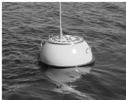
Figure 1 Photographies d'une bouée houlographe Waverider
