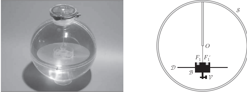
Figure 3 Plateforme stabilisatrice
