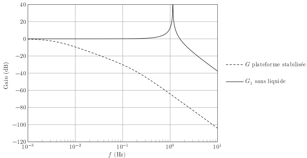
Figure 6 Diagrammes de Bode
