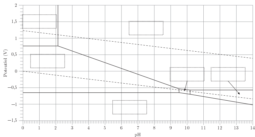
Figure A Digramme potentiel-pH du fer
