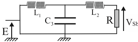
Figure 6 - Partie voie des basses
