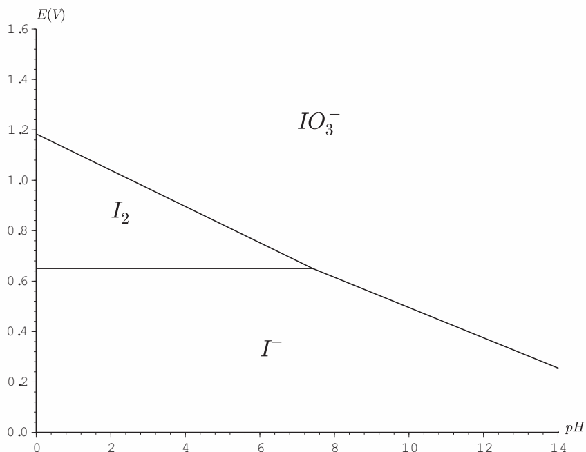
Figure 10 - Diagramme E-pH de l'iode
