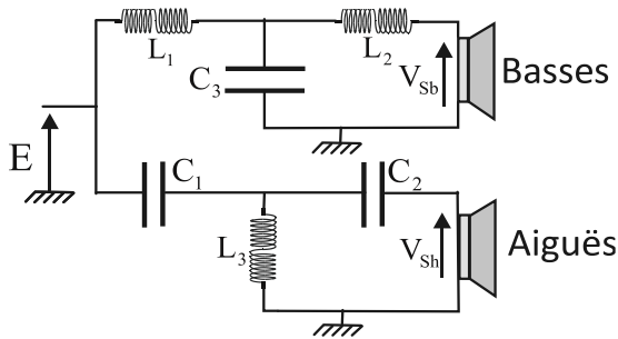
Figure 5 - Structure à deux haut-parleurs
