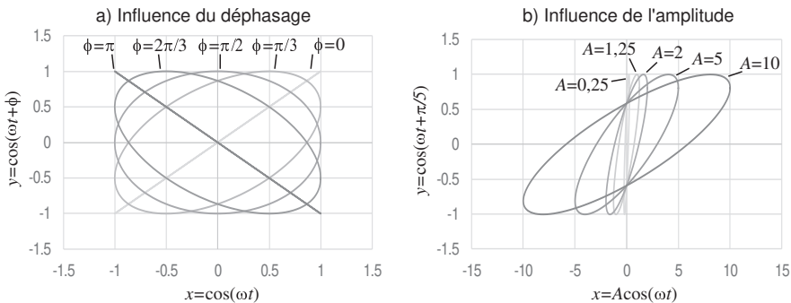
Figure 1 – Caractéristiques d'une ellipse pour une étude harmonique.
