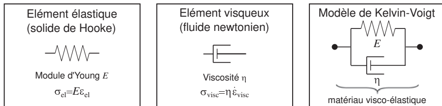
Figure 12 – Éléments de base pour la modélisation d'un matériau visco-élastique linéaire. De gauche à droite, sont représentés : un élément élastique (solide de HOOKE de module de YOUNG E ), un élément visqueux (fluide newtonien de viscosité \eta ) et une association en parallèle de ces deux éléments dans le modèle de KELVIN-VOIGT.
