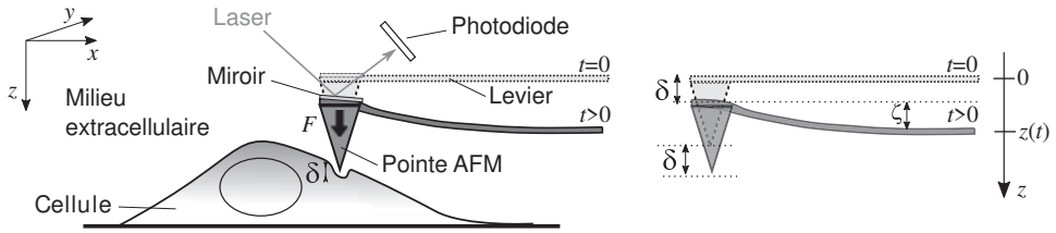
Figure 9 – Schéma de principe d'une expérience d'indentation d'une cellule par une pointe AFM. Les schémas représentent l'expérience vue de profil (axe vertical (Oz) dirigé vers le bas) à l'instant initial t = 0 où le levier est horizontal et à un instant t > 0 au cours de l'indentation où le levier est défléchi. Lorsque le levier est abaissé, la pointe indente la cellule et le levier fléchit. L'extrémité du levier est repérée par sa position verticale z . L'indentation \delta correspond à la position verticale de la pointe. La déflexion du levier est notée \zeta .
