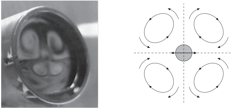
Figure 7 Photographie de la figure d'interférence (à gauche) et représentation schématisée associée du mouvement du cylindre (grisé) et des tourbillons générés (à droite)
