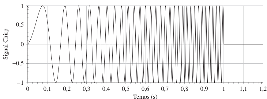
Figure 1 - Exemple de signal émis de type CHIRP
