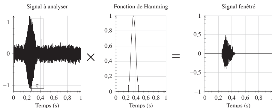
Figure 3 - Principe de la transformée de Fourier locale d'un signal : sélection d'une partie du signal autour de t = \tau en multipliant le signal à analyser par une fonction de Hamming
