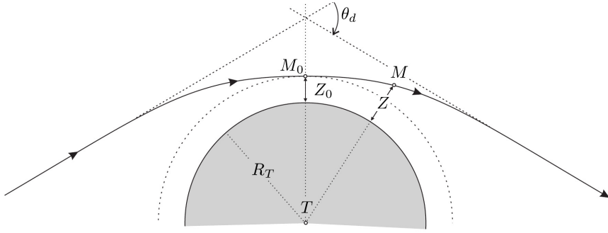
FIGURE 4 – Déviation d'un rayon lumineux par l'atmosphère terrestre.
