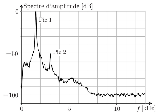
FIGURE 8 – Spectre d’amplitude d’un son sifflé tenu.
