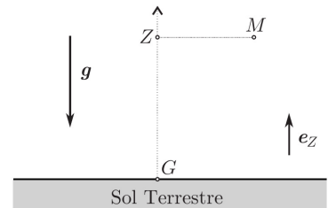
FIGURE 3 – Un point dans l'atmosphère terrestre.
