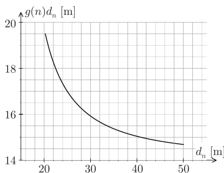
FIGURE 12 – g(n)d_n en fonction de d_n
