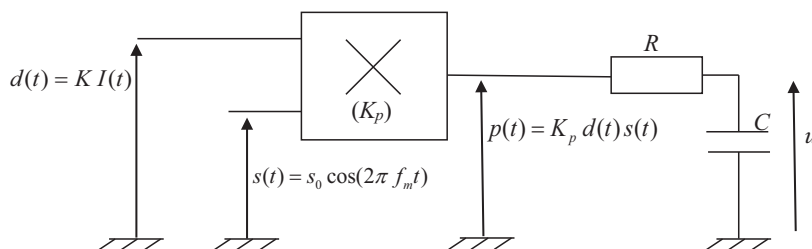
Figure 6 - Schéma du démodulateur
