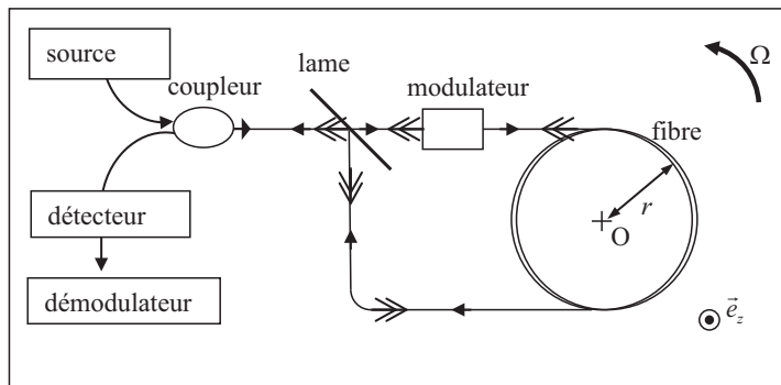
Figure 5 - Interféromètre de Sagnac à fibre optique
