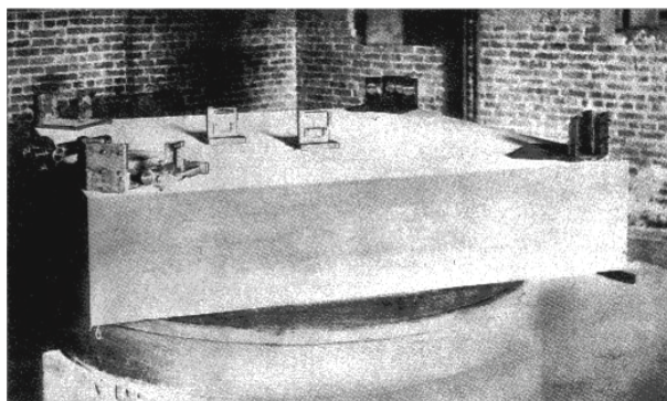
Photo 1 - L'interféromètre utilisé par Michelson et Morley en 1887
