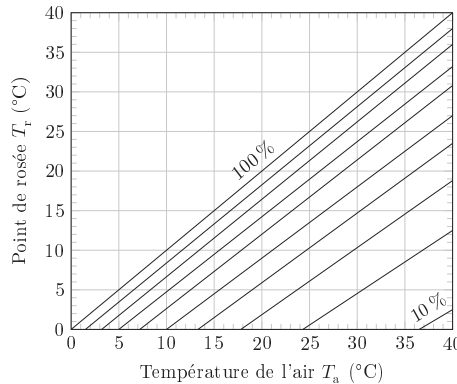
Figure 6 Point de rosée pour une humidité relative de 10 à 100 % par pas de 10 %
