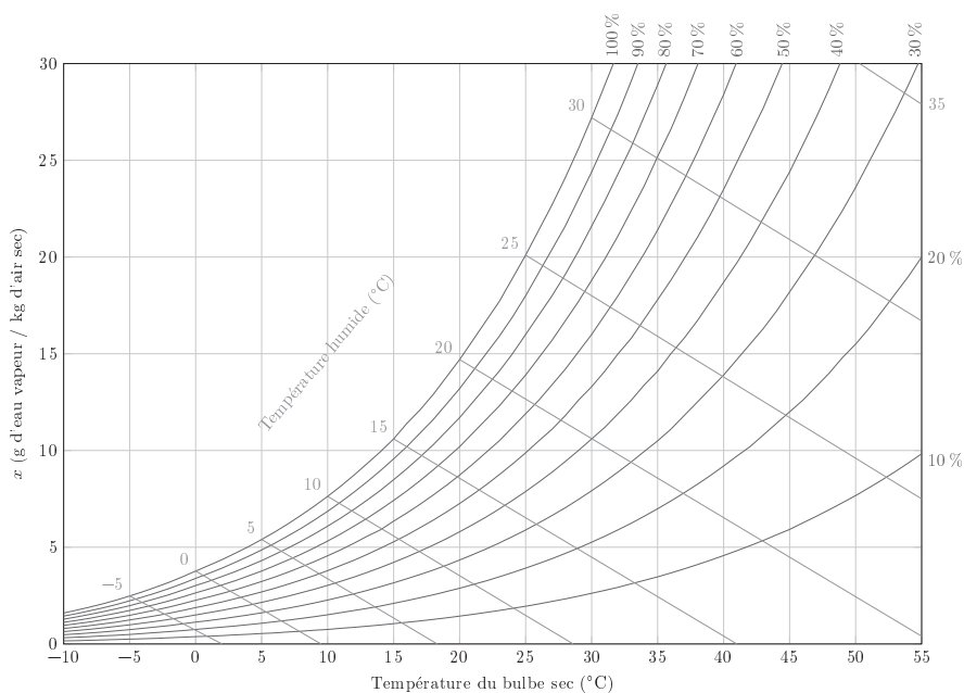
Figure A Diagramme psychrométrique
