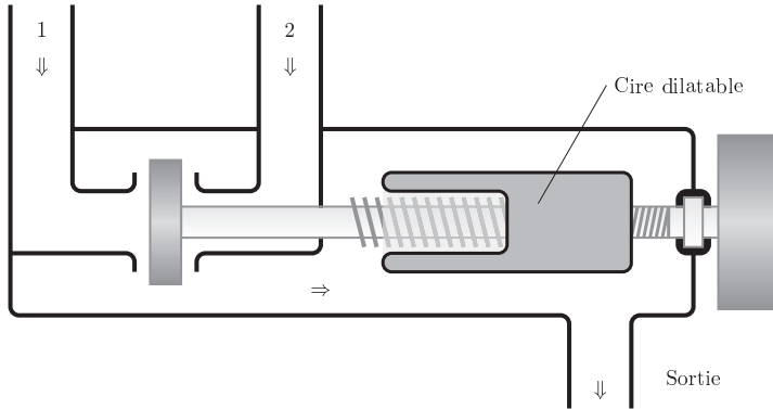
Figure 2 Mitigeur thermostatique schématique
