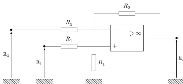
Figure 5 Montage soustracteur
