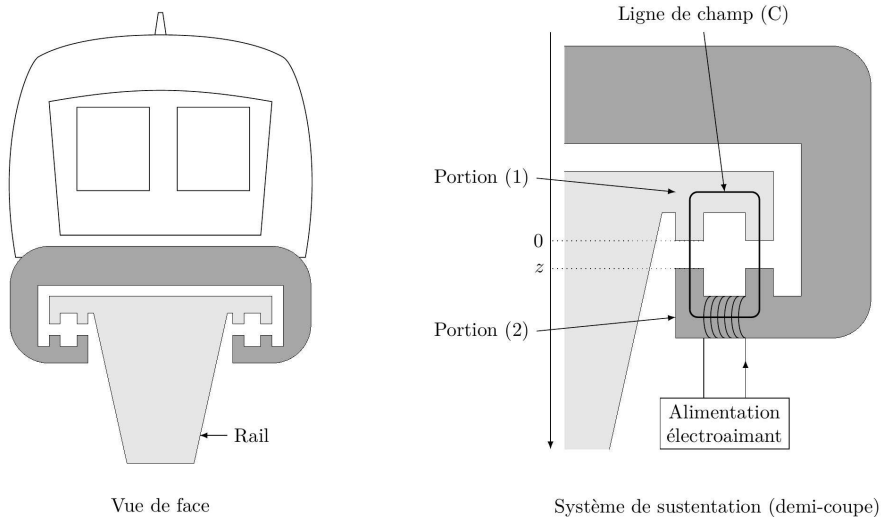
Figure 2 Transrapid et son système de sustentation
