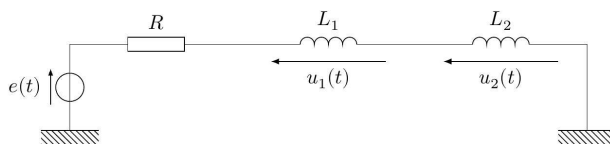
Figure 4 Alimentation du capteur
