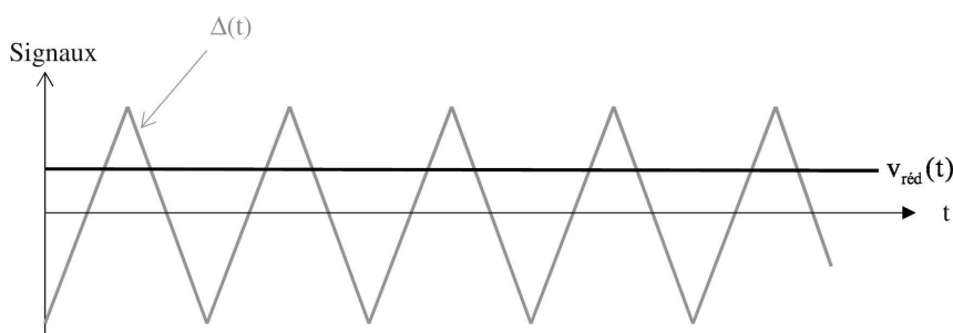
Figure 7 – Signaux pour l'élaboration du signal v_{\text{déc}}(t)
