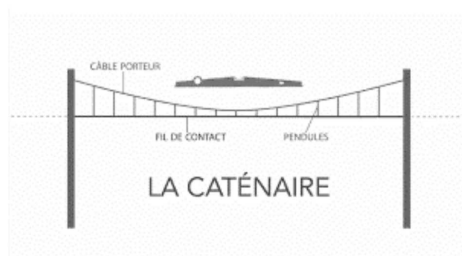
Figure 3 – Câble porteur et caténaire
