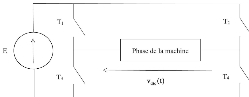
Figure 6 – Onduleur de tension
