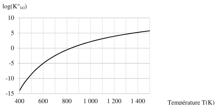
Figure 5 – Évolution de K^\circ_{(\text{a})} avec la température
