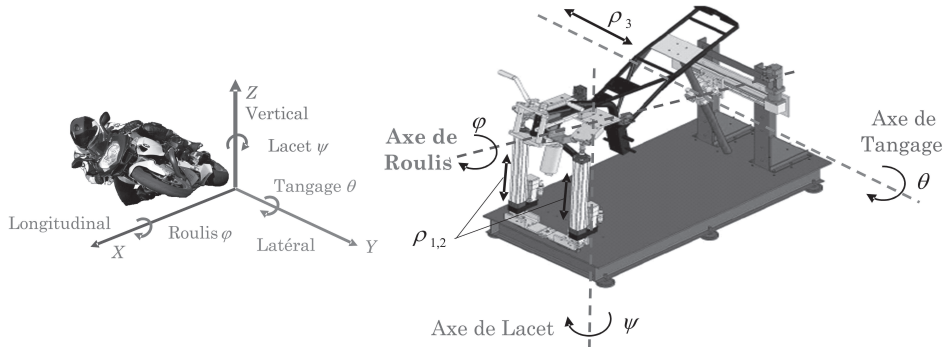
FIGURE 2 – Moto et plate forme. La rotation d'angle \psi autour de Z , dite de lacet, détermine la trajectoire ; la rotation d'angle \varphi autour de X , dite de roulis, définit l'inclinaison de la caisse lors d'un virage ; la rotation d'angle \theta autour de Y ( \theta_{\max} \approx 10^\circ ) décrit le tangage, rencontré notamment dans les phases d'accélération et de freinage. Le triplet (\varphi, \theta, \psi) est un exemple d'angles d'Euler.
