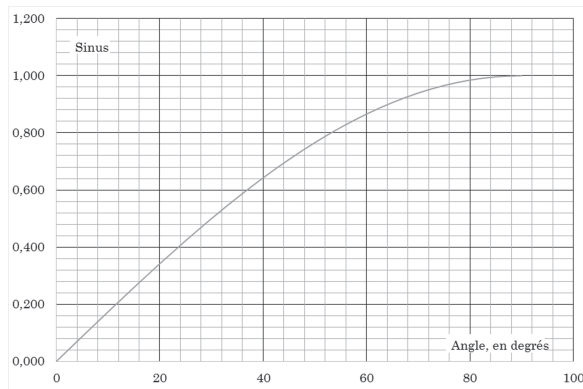
FIGURE 7 – Sinusoïde.
