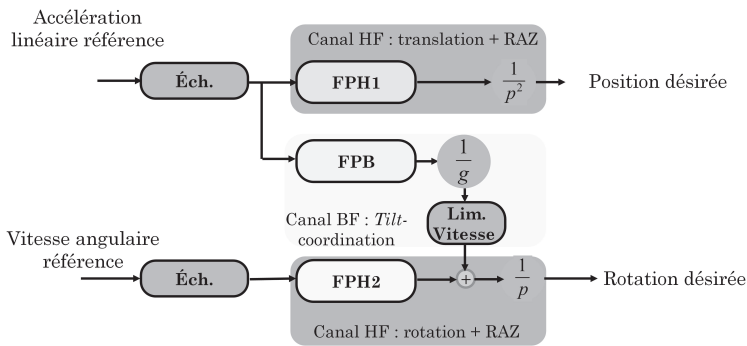
FIGURE 9 – Élément de l'algorithme de restitution du mouvement. Tilt = inclinaison. Noter la contribution du canal BF d'accélération à la position angulaire du simulateur.
