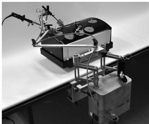
b - Robot Evolap avec simulateur abdominal
