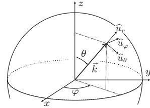
FIGURE 2 — Direction et sens du vecteur d'onde
