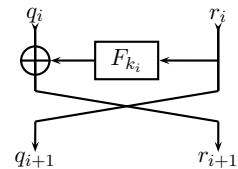
FIG. 1: Un tour de réseau de Feistel
