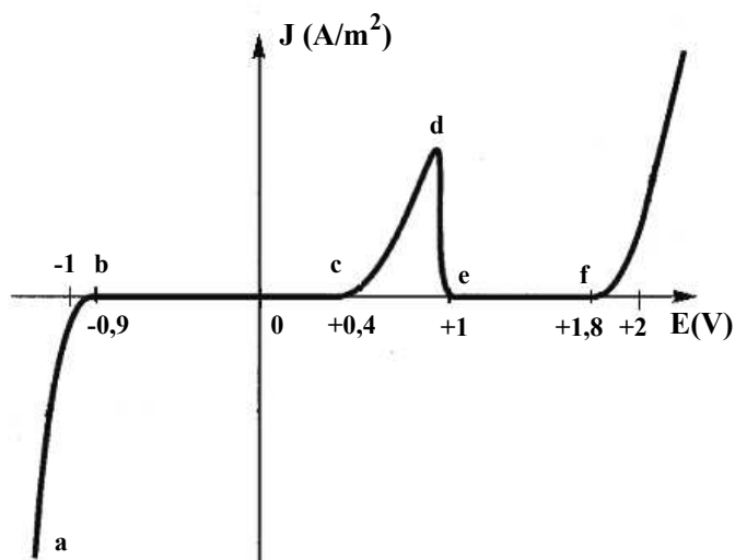
Figure 3 : courbe intensité-potentiel sur une électrode de plomb
