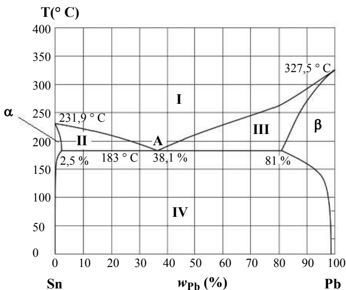
Figure 1 : diagramme de phase isobare solide-liquide du plomb-étain ( P^0 = 1 \text{ bar} )
