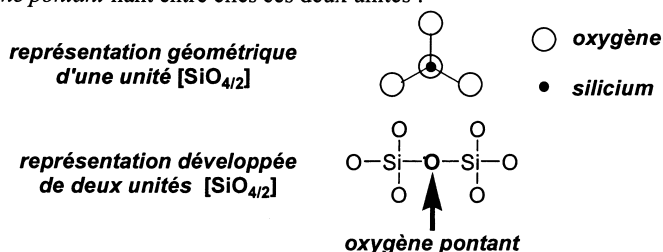
Figure 2 : Représentation d'unités tétraédriques de silicium
